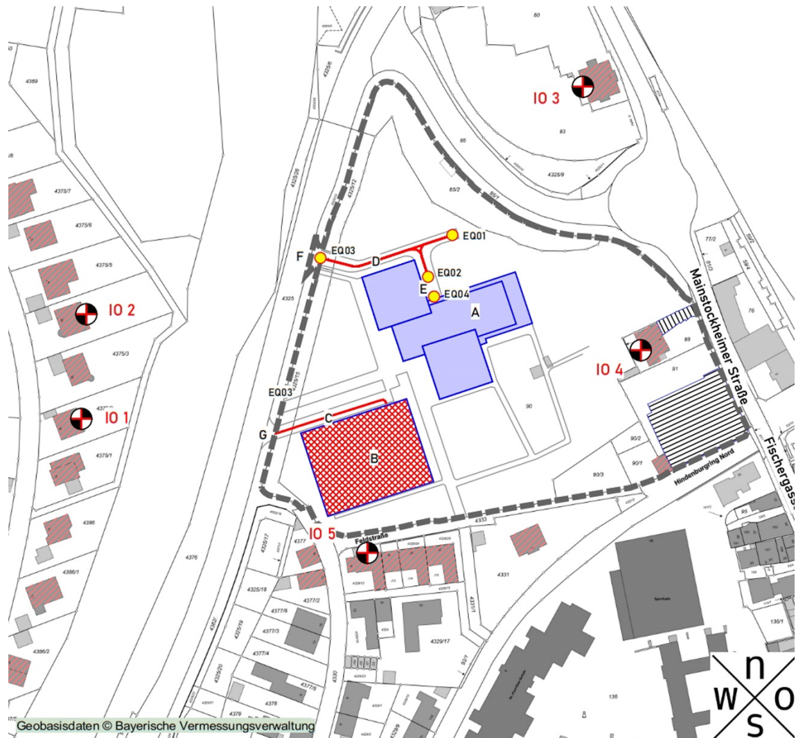
Abb.: Lage der berücksichtigten Immissionsort IO 1 bis IO 5, Wolfgang Sorge Ingenieurbüro für Bauphysik 2020
